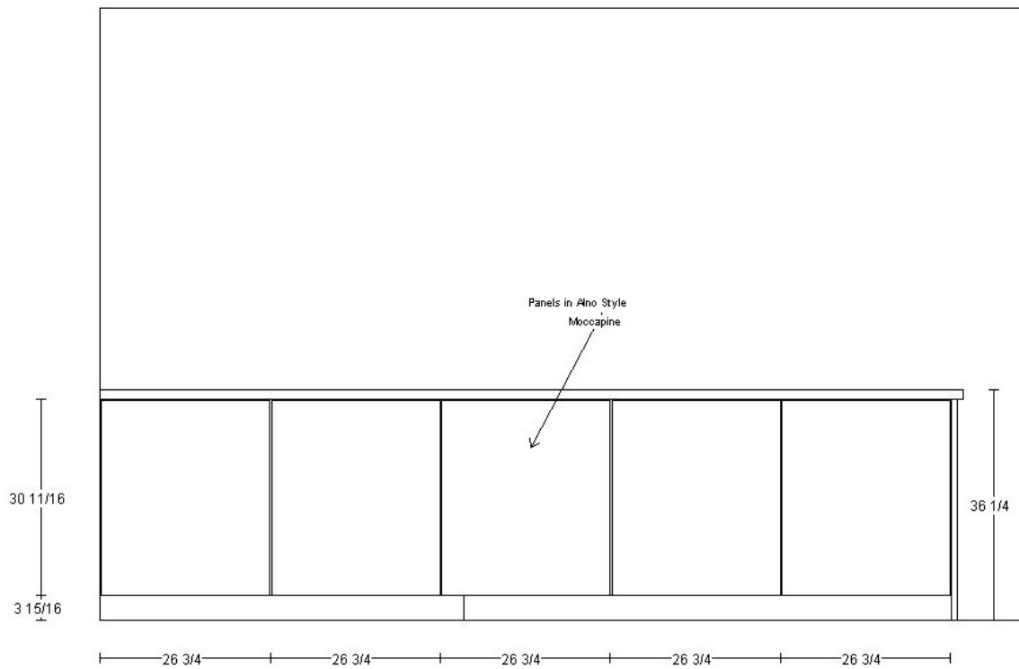
Elevation E
